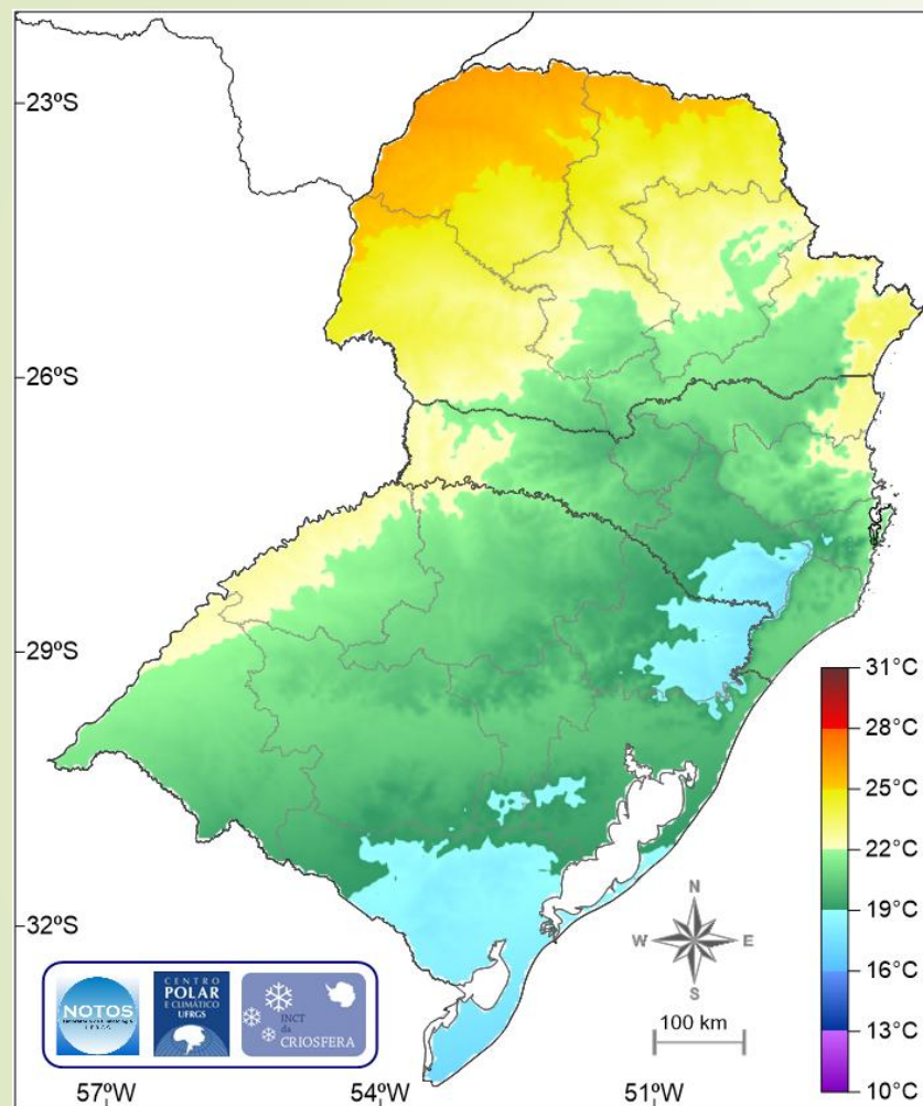
Climatologia 1981-2010 (CRU/SRTM)
