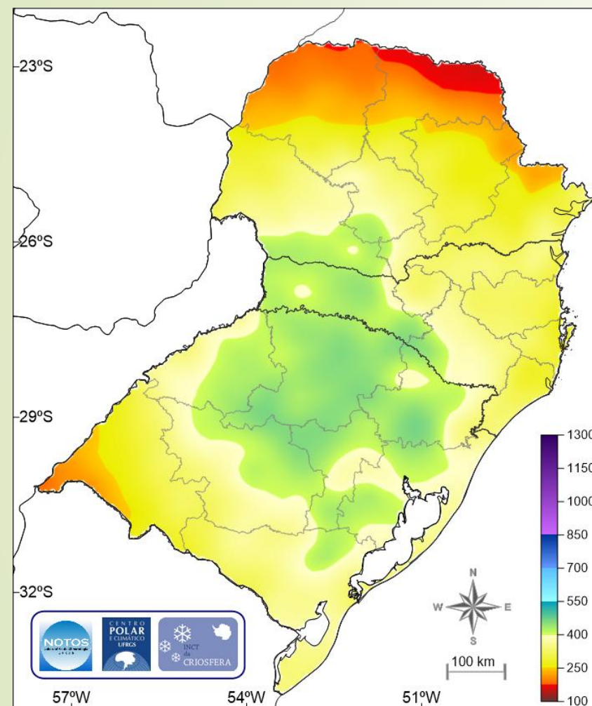
Climatologia 1981-2010 (GPCC)
