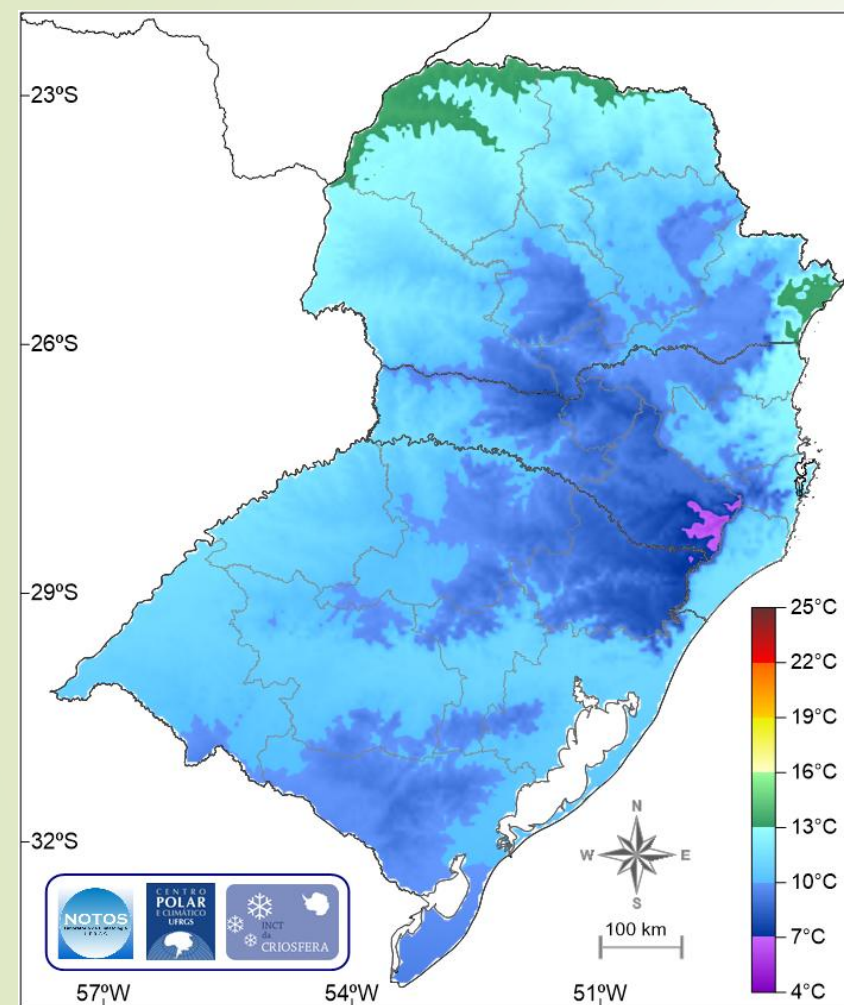
Climatologia 1981-2010 (CRU/SRTM)
